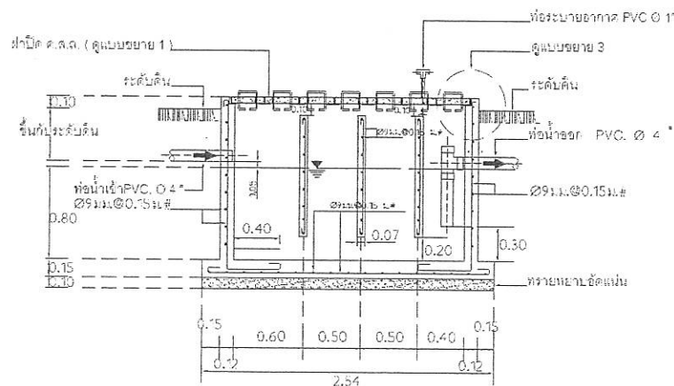
แปลนภาพตัดขวางตามแนว A-A ของบ่อดักไขมันแบบคอนกรีตเสริมเหล็ก
