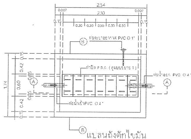
แปลนภาพด้านบนของบ่อดักไขมันแบบคอนกรีตเสริมเหล็ก
